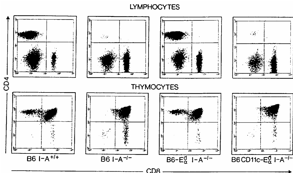
Figure 1 : Marquage des splénocytes et les thymocytes des souris C57BL/6 (B6), B6 I-A -/- , B6.E \alpha^d I-A -/- et B6.CD11cE \alpha^d I-A -/- avec anti-CD4 et anti-CD8.
