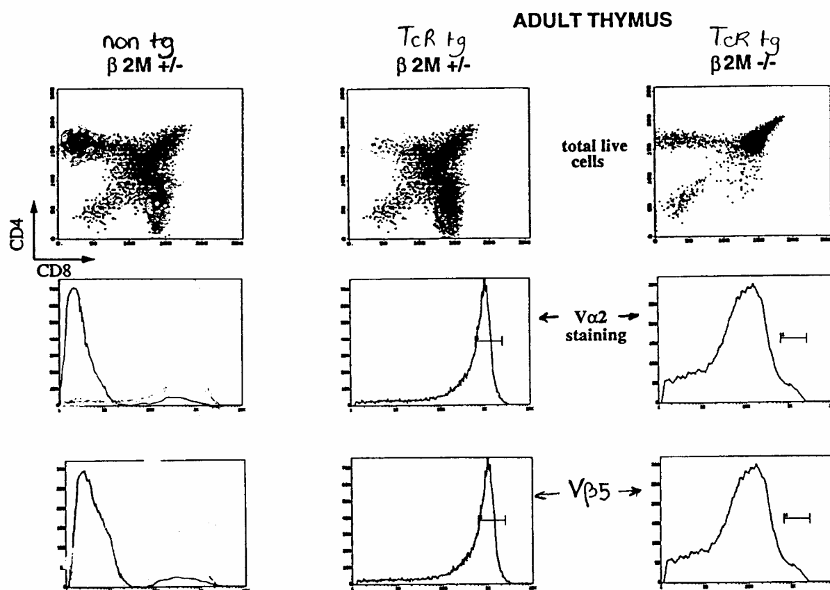
Figure 2 : Marquage des thymocytes de souris non transgéniques \beta 2m^{+/-} (non tg), TcRtg \beta 2m^{+/-} et TcRtg \beta 2m^{-/-} avec des anticorps anti-CD4, anti-CD8, anti- V\alpha 2 et anti- V\beta 5 .
